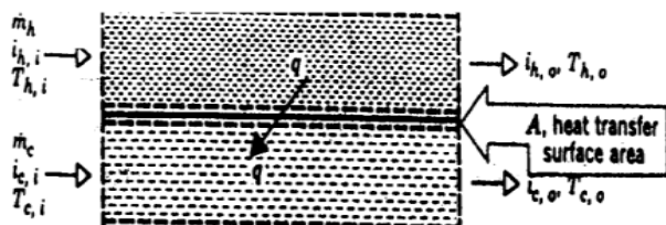
Gambar 1. Skematik alat penukar panas
