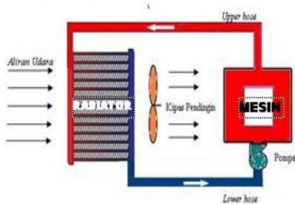
Gambar 2. Skematik radiator
