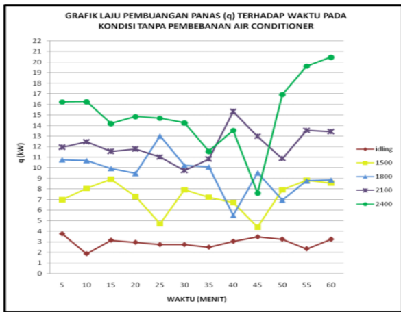
Gambar 4. Grafik laju pembuangan panas terhadap waktu tanpa beban AC
