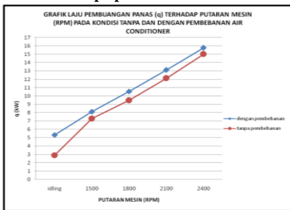
Gambar 6. Grafik laju pembuangan panas rata-rata terhadap rpm mesin
