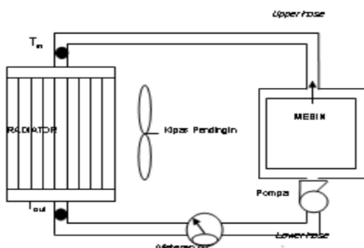
Gambar 3. Skematik pengujian radiator
