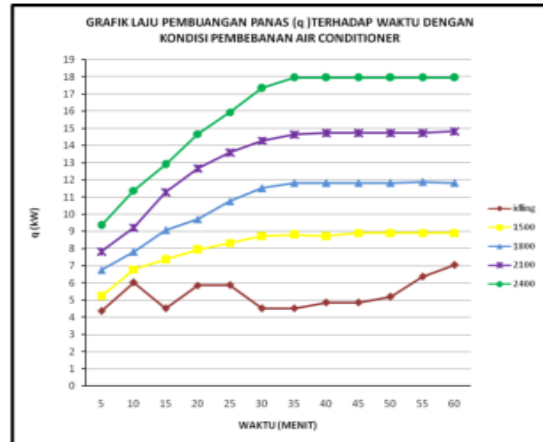
Gambar 5. Grafik laju pembuangan panas terhadap waktu dengan beban ac
