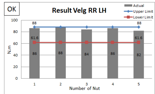
Gambar 32. Grafik Result Velg RR LH
