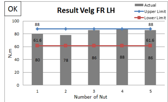
Gambar 31. Grafik Result Velg FR LH
