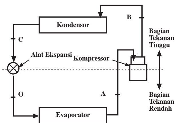
Gambar 1. Siklus refrigerasi Standart
