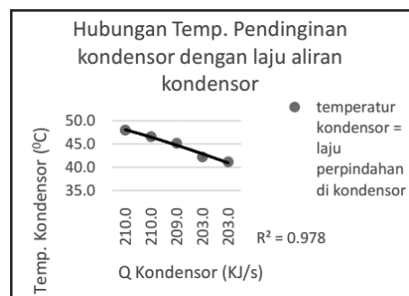
Gambar 3. Pengaruh laju pelepasan kalor kondensor terhadap temp. Kondensor.
