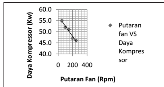
Gambar 5. Pengaruh putaran fan kondensor terhadap daya kompresor.
