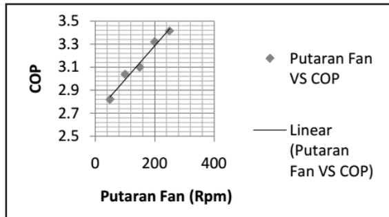
Gambar 4. Pengaruh kecepatan putar terhadap nilai COP.
