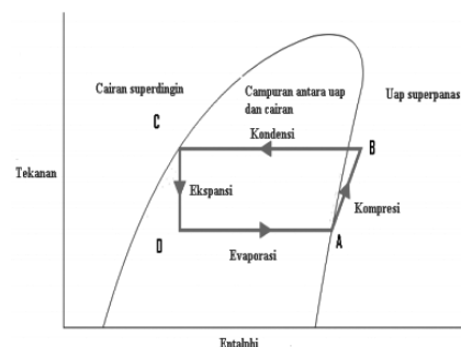
Gambar 2. Diagram P-h siklus kompresi uap
